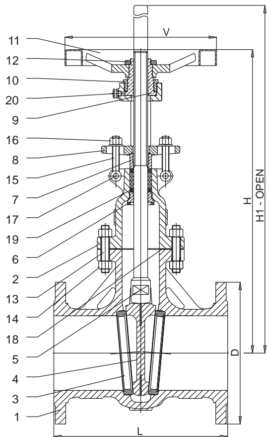
FIG. 1190 - DIN PN 16: Face to Face F5
