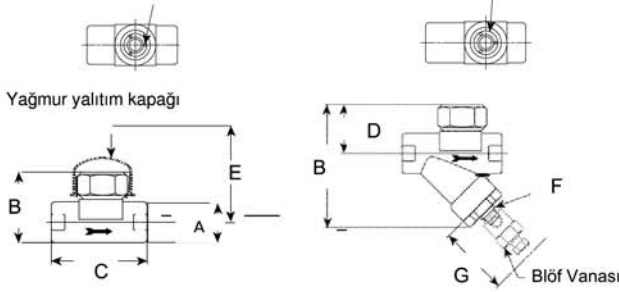
3 Tahliye kanallı dizayn
