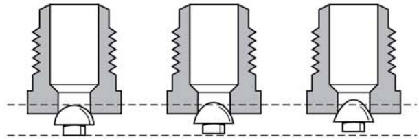
Armstrong ters kovalı kondenstopun küresel supabı aşınma oluştuğunda bile sit içinde daha derine oturarak tam sızdırmazlığı sağlar .
